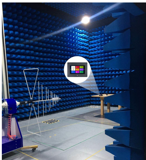
图 6-5 辐射测试图
