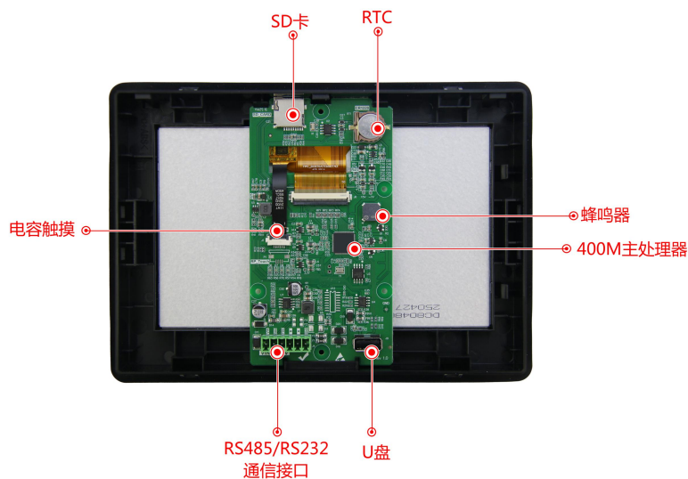
图 1-2 硬件配置图
