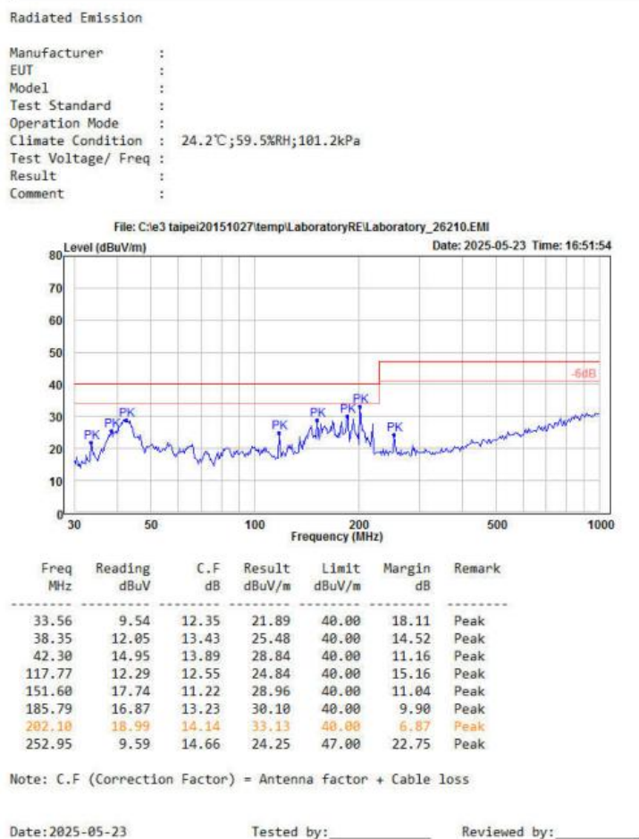
图 6-7 辐射测试垂直方向
