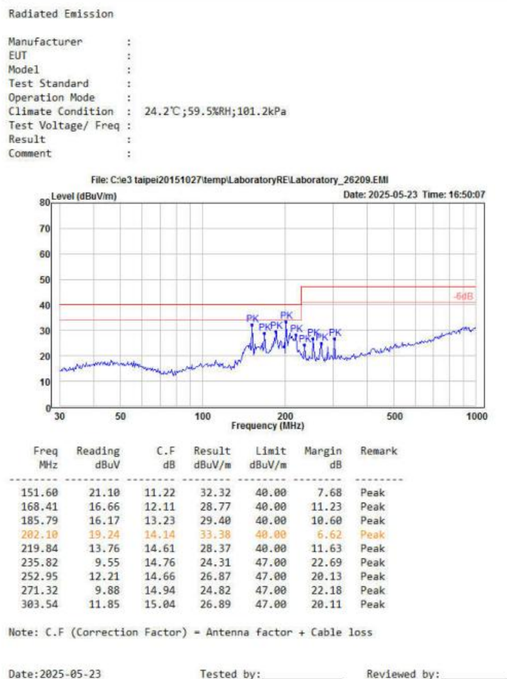
图 6-6 辐射测试水平方向
